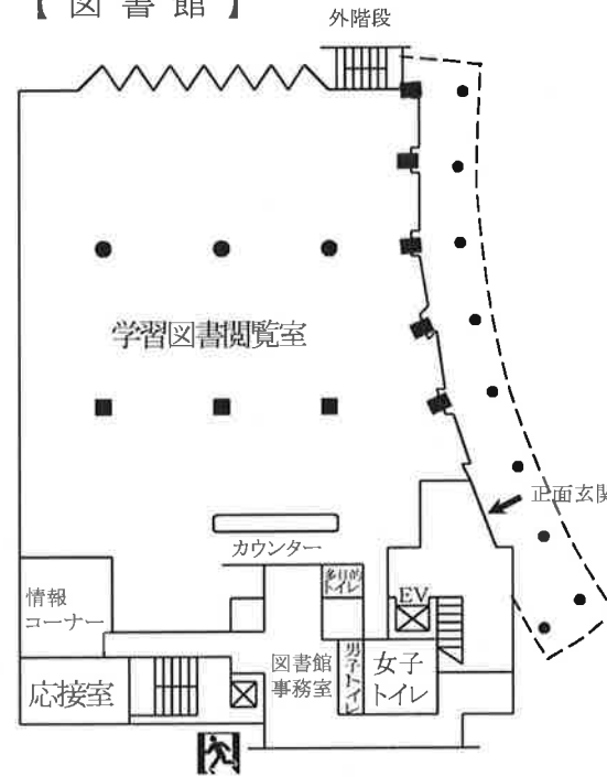
図書館1階
